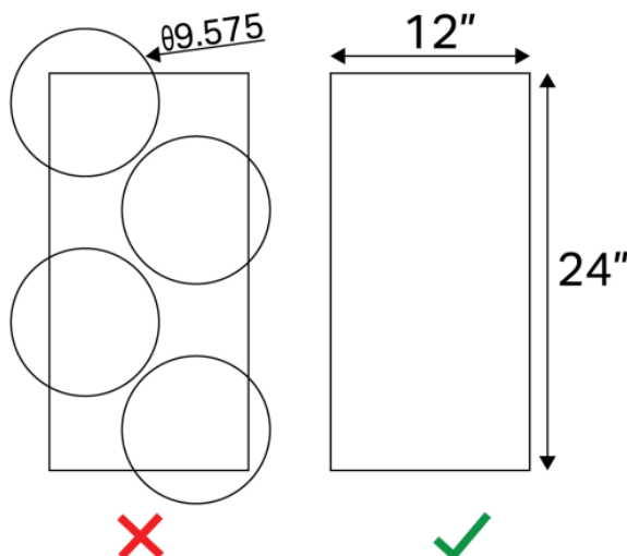
图 23 自制塑料件须可容纳于单块 12" × 24" 的塑料板内
