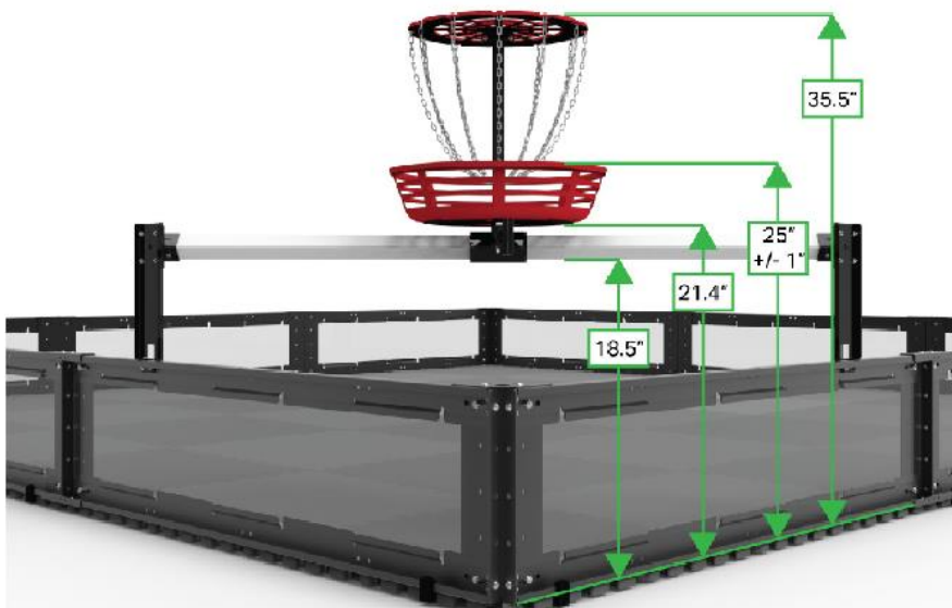
图 20 高筐的垂直尺寸
